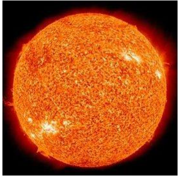
太陽 ☉
