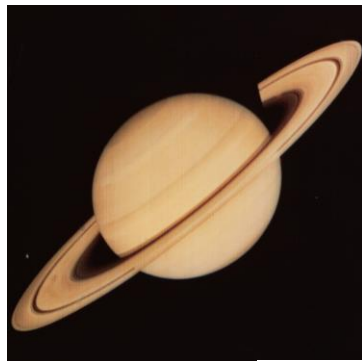
土星 ♄
